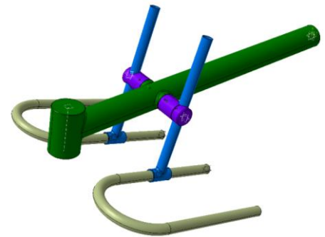
Figure 1 - modélisation 3D cale pieds existant (GROUPE 1)
